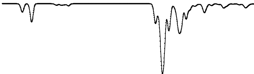
IR Spectrum of 5
