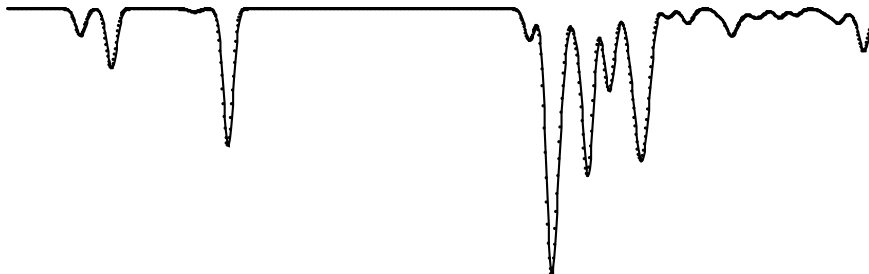
IR spectrum of 6
