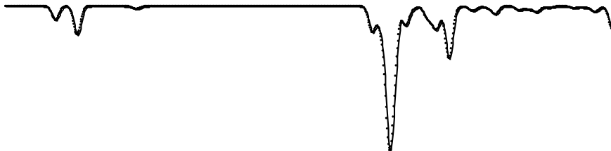
IR Spectrum of 5
